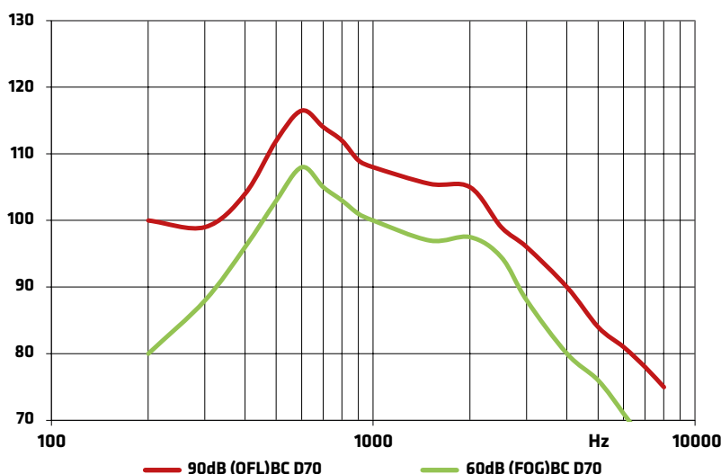
dB OFL90 Ausgangskraftpegel, FOG(60) akusto-mechanischer Kraftpegel
